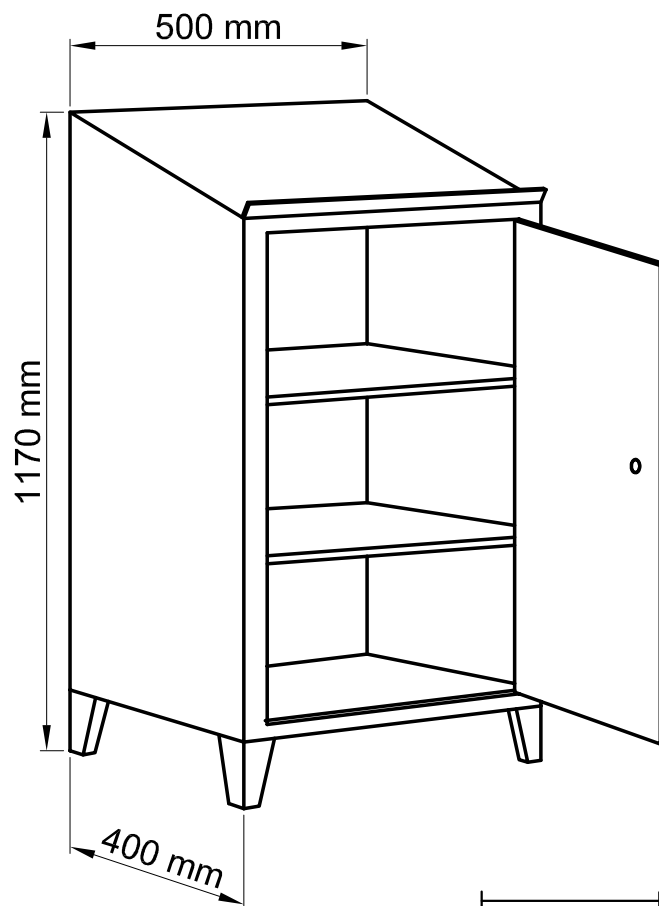
MODELLO CON PIEDINI CON RIPIANI
