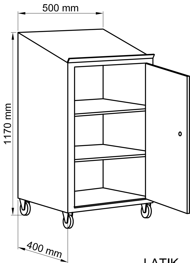
MODELLO SU RUOTE CON RIPIANI
