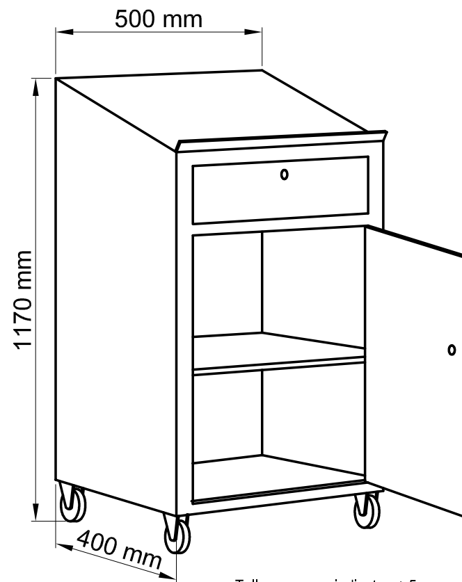
MODELLO CON CASSETTO CON RIPIANO
